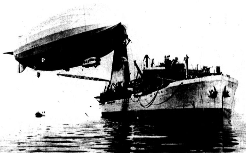
Das Luftschiff Los Angeles (Z. R. III) bei dem ersten Versuch, auf offenem Meer zu verankern
