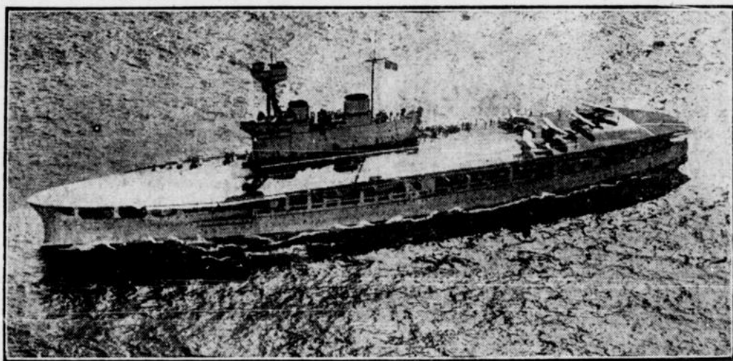
„Eagle“ hatte eine Wasserverdrängung von 22.672 Tonnen und war ursprünglich als Linienschiff vorgesehen, dann aber in einen Flugzeugträger umgebaut und in der Zwischenzeit mehrfach baulich verändert worden. Zum Schutz gegen U-Boote hatte das Schiff besondere Torpedowulste erhalten. Seine Bewaffnung bestand aus neun 15,2-Zentimeter-Geschützen, vier 10,2-Zentimeter-Luftabwehr-Geschützen, vier 4,7-Zentimeter-Geschützen, acht 4-Zentimeter-Flak-Geschützen und 13 Flak-MGs. In Friedenszeiten hatte das Schiff 21 Flugzeuge an Bord; die Besatzung betrug 750 Mann.
