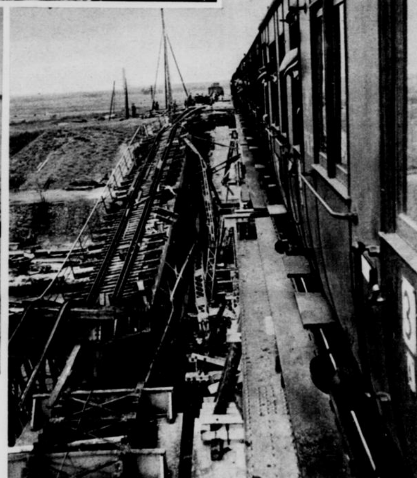
Zum erstenmal über die neue Warthebrücke Am 2. Oktober 1939, nachmittags 4 Uhr, fuhr der erste Personenzug über die neue Warthebrücke bei Sieratz auf der Strecke Lodz—Breslau. Links ist noch die von den Polen bei ihrem Rückzug zerstörte alte Eisenbahnbrücke zu sehen Aufn. Associated Press
