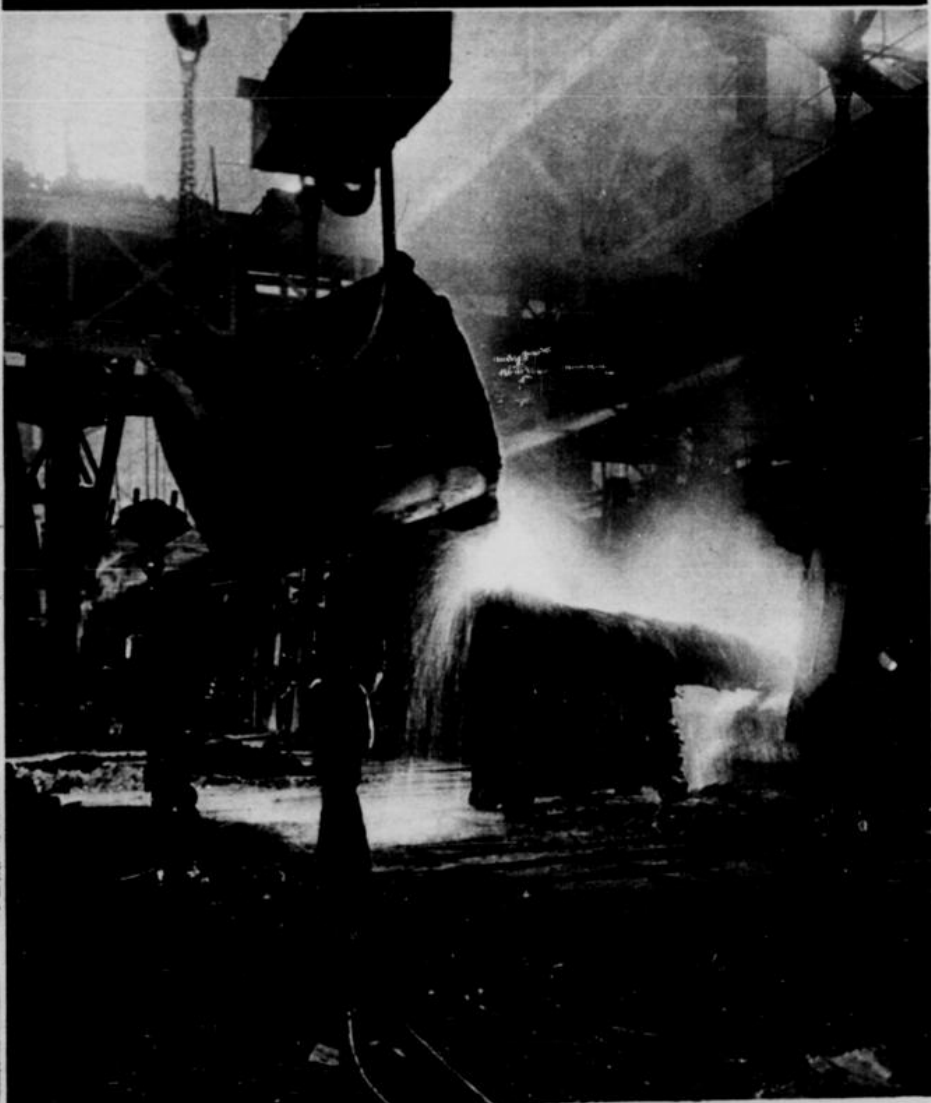
Einguß von Roh Eisen in den Siemens-Martin-Ofen
