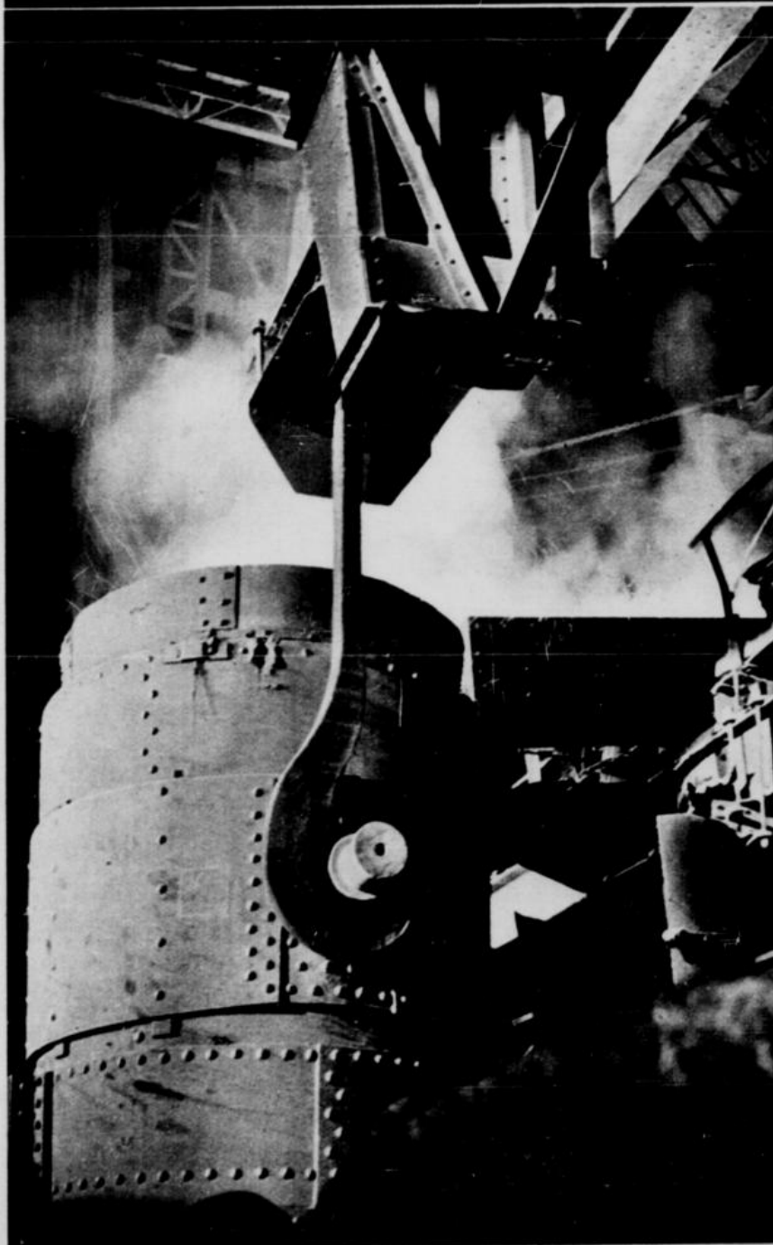
Einguß von Roh Eisen in den Siemens-Martin-Ofen
