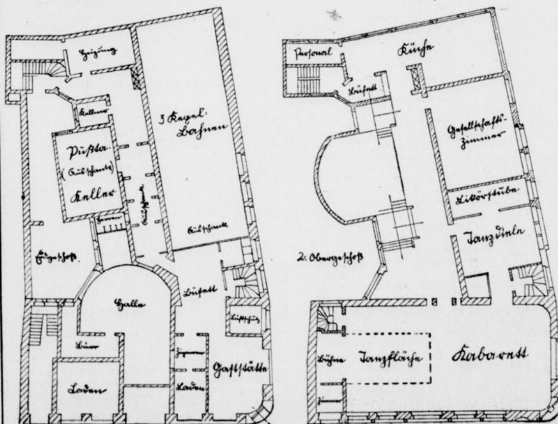
Der Grundriß für das Untergeschloß und das zweite Obergeschloß
