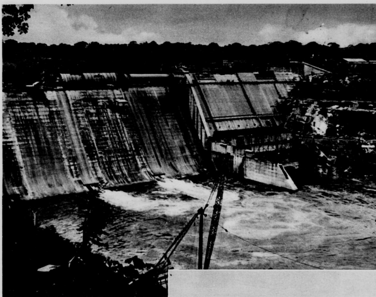
Der Maddendamm. Das neue Stauwerk des Kanals. Während in niederschlagsreichen Jahren der Gatunsee genügend Wasser besitzt, um die Schiffschiffahrt und die Operationen der Schleusen zu gewährleisten, tritt in trockenen Jahren eine unangenehme Wasserarmut ein, der man jetzt durch den Bau einer riesigen Stauanlage begegnen will. Der Maddendamm enthält ca. 500.000 cbm Zement. Das durch ihn entstehende Reservoir wird 22 Billionen Kubikfuß Wasser fassen. Aufn. Welt Rundschau
