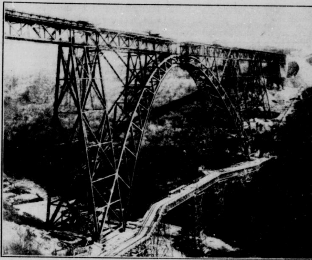
Die Brücke kurz vor Bogenschluß Ende März 1897 und die 30 Meter hohe provisorische Brücke, von der aus durch eine Drahtseilbahn der Baumaterialien-Transport geleitet wurde.
