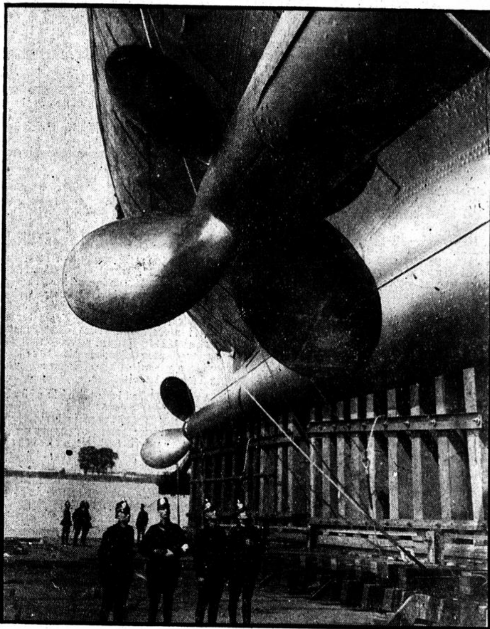
Eine der riesenhaften Schrauben des Lloyd-Dampfers „Bremen“, dessen Stapellauf soeben in Bremen stattfand.
