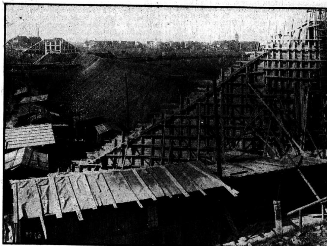
Widerlager bei der Brücke Reichsbahn-Durchlaß, Goldhammer Bach. Im Hintergrund rechts der Turm einer Kirche in Hordel.
