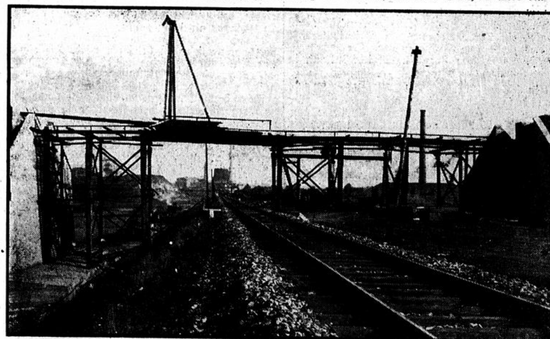
Montage-Gerüst für die Brücke über die Reichsbahn.
