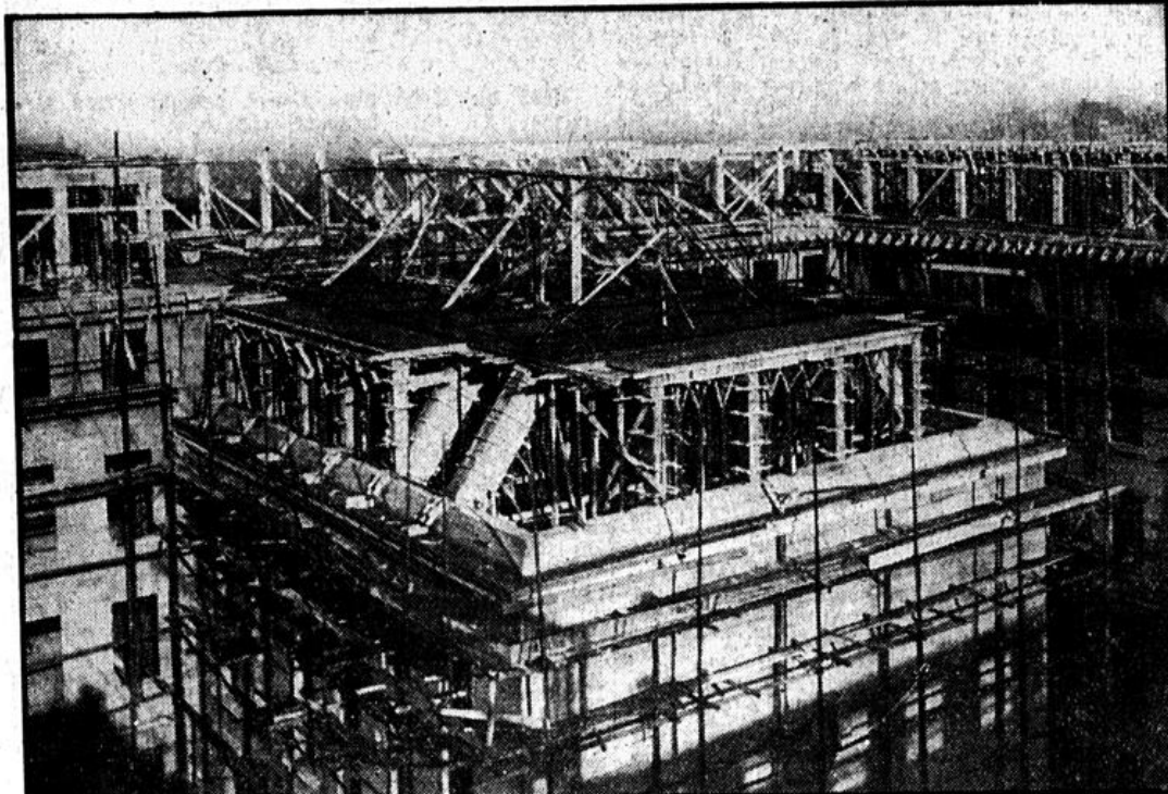
Der Neubau unseres Rathauses hat in den letzten Tagen erhebliche Fortschritte gemacht. Die Zimmerleute, die vor wenigen Tagen daran gegangen waren, den Dachstuhl zu errichten, haben ihre Arbeit, wie unser Bild zeigt, nahezu vollendet.
