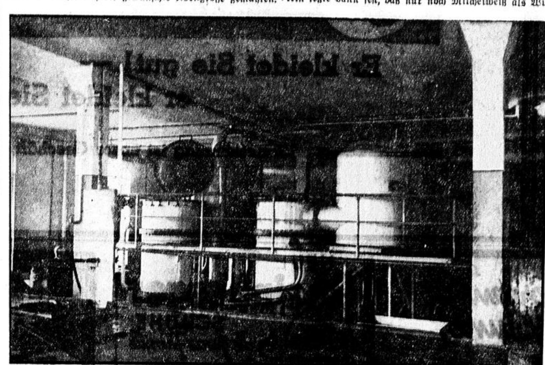
In diesen Vacuumbehältern wird die Magermilch unter Schonung ihrer Bestandteile kondensiert.
