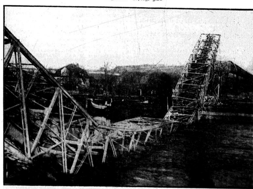
Der Sturz einer Drahtseilbahnbrücke in die Saale
