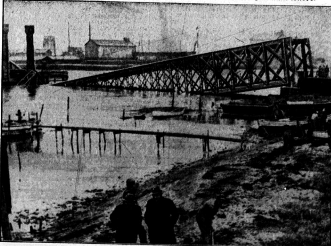
Die von einem englischen Dampfer gerammte Brücke im Masnedé-Sund (zwischen den Inseln Seeland und Masnedé) rügte ein, wodurch diese wichtige Eisenbahnlinie unterbrochen wurde. Man sieht hier die eingestürzte Brücke, die jedoch bis Weihnachten wieder hergestellt sein wird. (Presse-Photo-M.)
