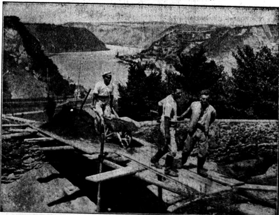
Auf dem Loreley-Felsen wird gegenwärtig von Arbeitsdienstmannern ein Thingplatz errichtet. Das Bild zeigt die Arbeitsmänner bei der Arbeit. Im Hintergrund der Rhein. (Presse-Bild-Zentrale-M)
