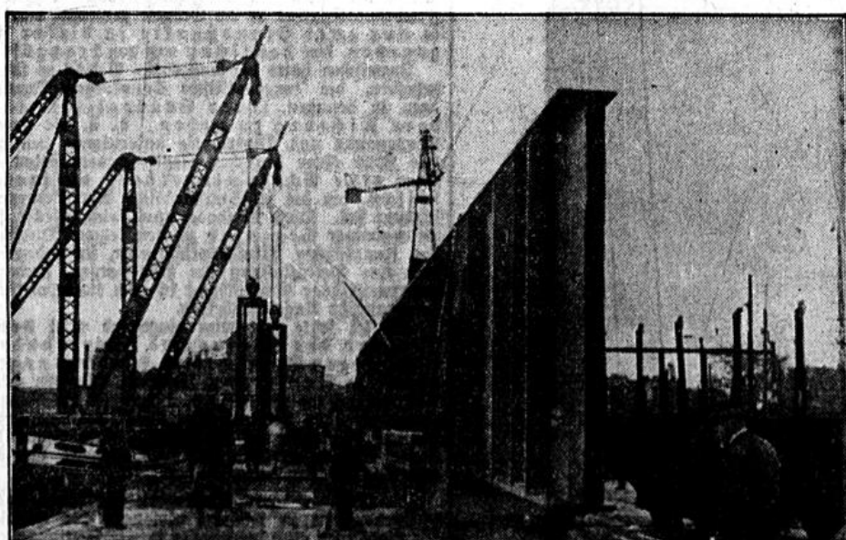
Der größte elektrisch geschweißte Brückenträger der Welt.
