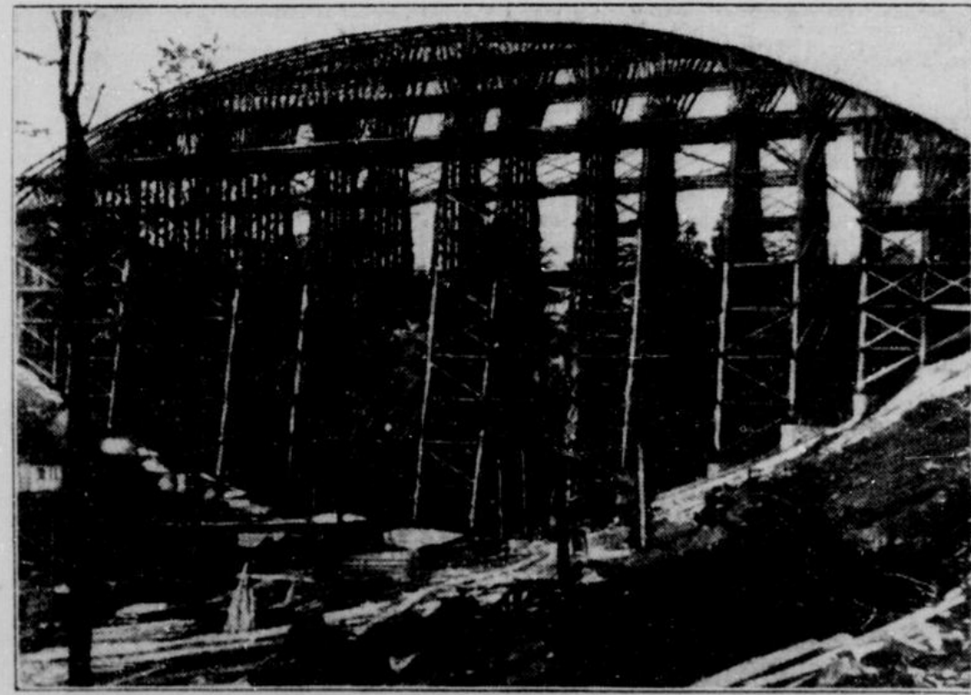
Deutschlands größte Bogenbrücke aus Eisenbeton im Bau
