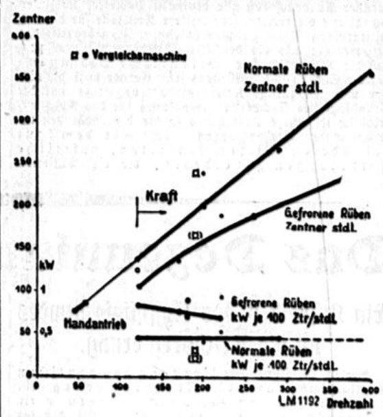
Diagramm des neuen Flachegelrübenschniders von Stille mit Stiftenmessern.
