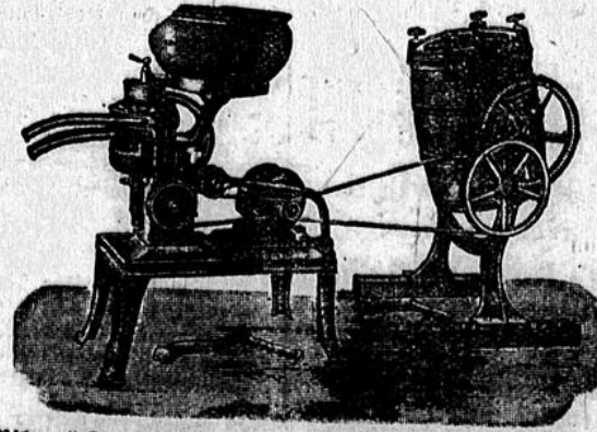
Milena-Zentrifuge mit Teller-Einfaß, 400—600 Liter fähig. Leistung, für unmittelbaren elektrischen Antrieb, verbunden mit einer „Miele“-Sturzbuttermaschine Wo die Verhältnisse es gestatten, sollte man unbedingt elektrisch entrahmen und auch elektrisch buttern. Wir glauben, sagen zu dürfen, daß in einigen Jahrzehnten in Deutschland die elektrische Entrahmung das Normale und die Handentrahmung die Ausnahme sein wird. In elektrischen Zentrifugen und Butter-
