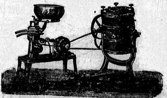
Milena-Zentrifuge mit Teller-Einfaß, 160—220 Liter fähig. Leistung, für unmittelbaren elektrischen Antrieb, verbunden mit einer „Miele“-Sturzbuttermaschine
