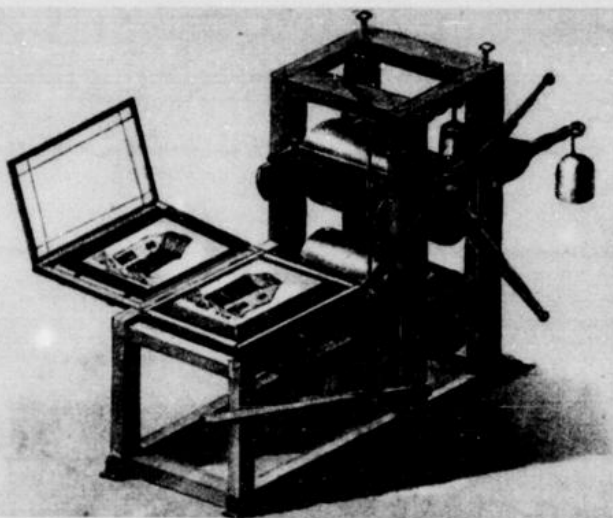
Die Druckmaschine Senefelders
