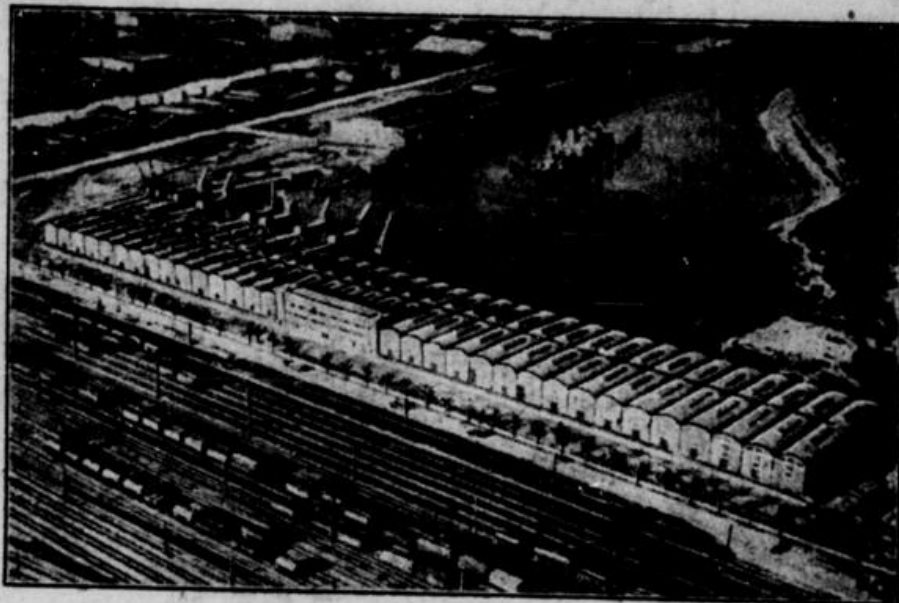
Dieser Tage ist im Südwesthafen in Hamburg der neue Kaischuppen 39 fertiggestellt worden. Der 331 Meter lange und 50 Meter breite Eisenbetonschuppen hat nur eine Reihe Zwischenstützen; interessant ist die neuartige Tonnendach-Konstruktion der Anlage.
