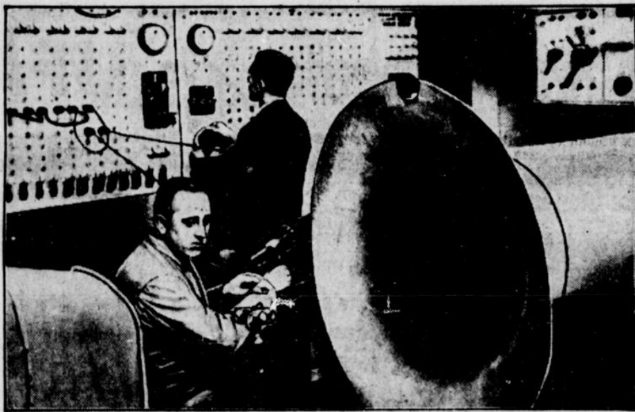
In dem vor kurzem eröffneten neuen Heim der Meteorologischen Versuchsanstalt der Deutschen Seewarte in Hamburg befindet sich ein Windkanalraum, in dem zu Forschungszwecken Windstärken bis zu 40 Meter in der Sekunde erzeugt werden können.
