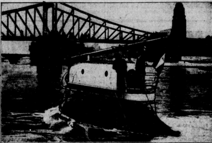
Das neuartige Boot auf dem Main bei Frankfurt; es hat einen verstellbaren Tiefgang bis zu 3,80 Meter und kann somit praktisch nicht kentern. Das von dem Deutschen Albert Sigg konstruierte Boot hat neben einem Motor ein Segel von 28 Quadratmeter.
