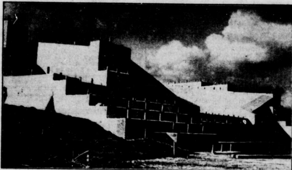
Die bizarre Konstruktion eines Widerlagers zur Ueberführung des Mittellandkanals über die Elbe bei Magdeburg. Die Bauarbeiten an dem Mittellandkanal schreiten trotz allen wirtschaftlichen Schwierigkeiten ruhig vorwärts.
