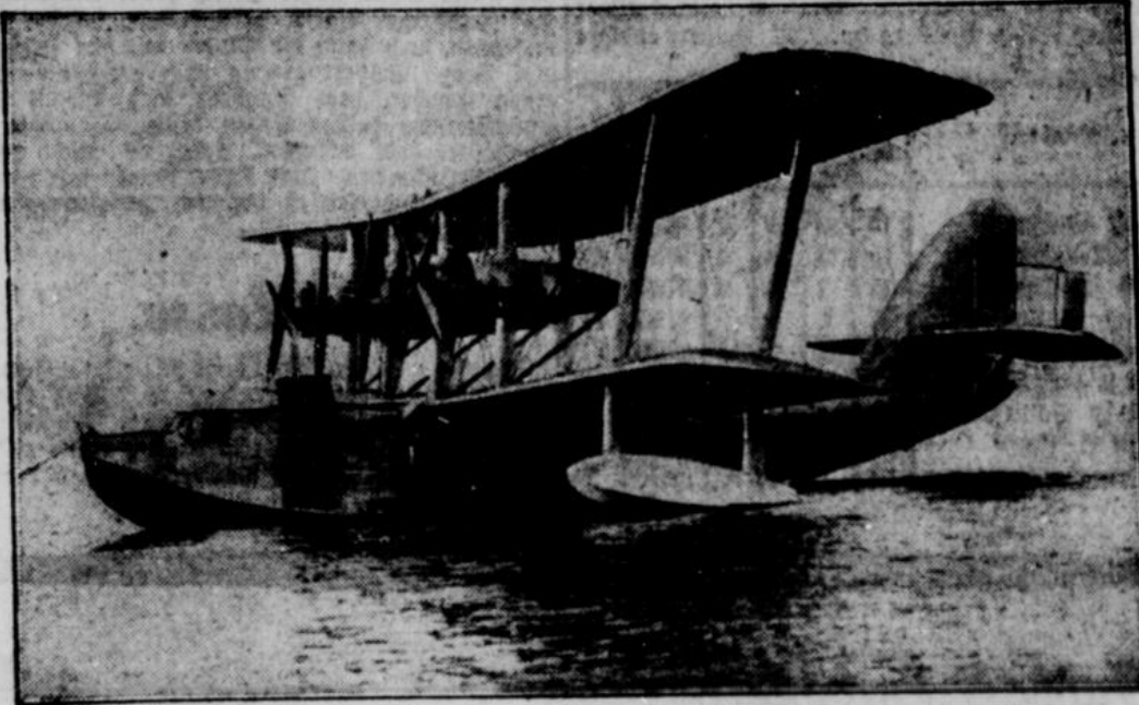
In Rochester (England) ging dieser Tage das erste von drei Großflugbooten vom Stapel, die den regelmäßigen Flugverkehr zwischen England und Süd-Afrika aufnehmen sollen. Es ist das größte bisher in England gebaute Flugboot und kann außer der Besatzung 16 Passagiere und 32 Doppelzentner Post und Fracht aufnehmen.
