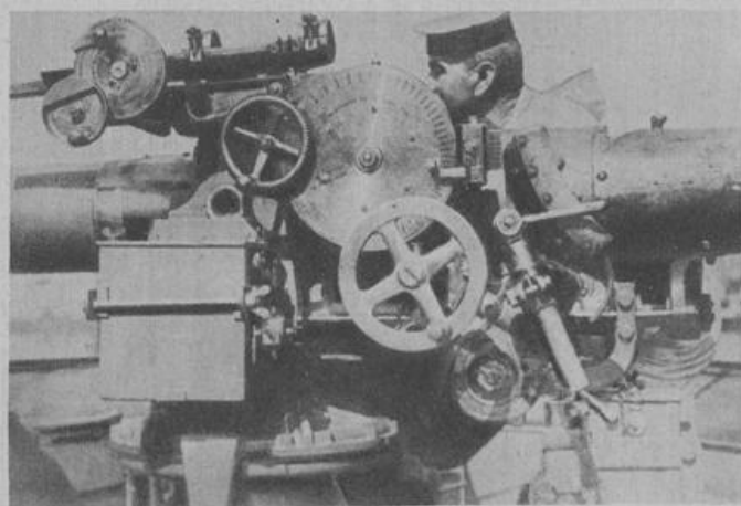
Richt- und Zielvorrichtung einer Schiffskanone, die sich an Bord englischer Dreadnoughts befindet
