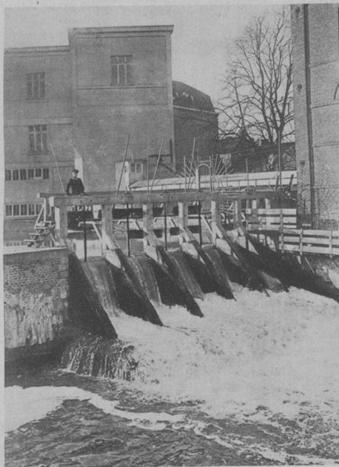
Das Elektrizitätswerk in Vitré en Artois, das von deutschen Soldaten betrieben wird. Phot. Braemer
