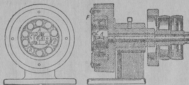
Querschnitt der Danton'schen Siefenmaschine. Längsschnitt.
