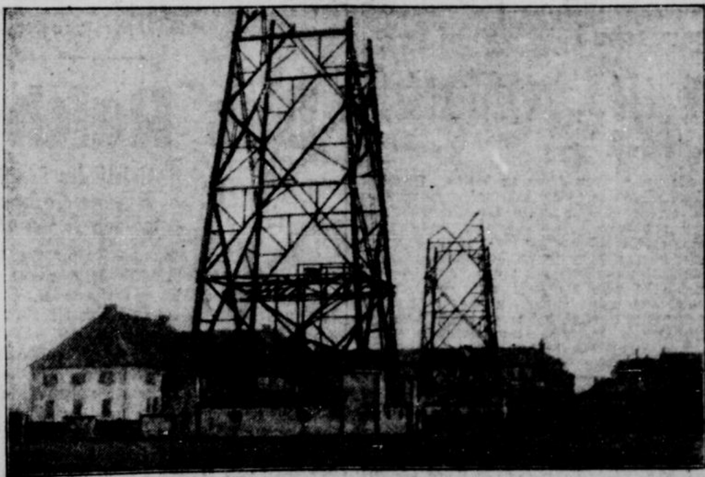
Durch den heftigen Sturm, der am Sonntagmorgen über München tobte, stürzten die beiden Funktürme der Deutschen Stunde in Bayern bei Stadelheim um. Die Türme wurden in einer Höhe von etwa 25 Meter umgebrochen. Glücklicherweise sind Sendebäude und Maschinen nicht beschädigt worden; desgleichen sind Verletzte nicht zu beklagen.
