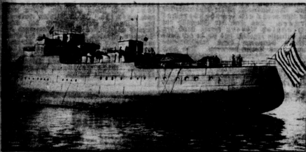
Auf der Germania-Werft in Kiel lief am Dienstag die für den amerikanischen Milliardär Vanderbilt-Newyork erbaute Luxus-Motor-Jacht „Alva“ vom Stapel. Das Fahrzeug hat eine Wasserverdrängung von 3500 Tonnen, besitzt zwei Viertakt-Krupp-Dieselmotoren von 4200 PS, ist zirka 90 Meter lang und zirka 15 Meter breit.
