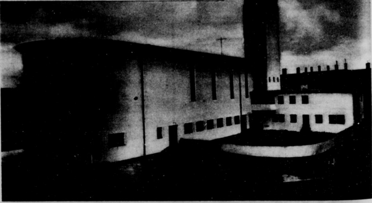
Die erste Eisenbetonkirche Deutschlands Die Petri-Nikolai-Kirche in Dortmund stellt ein Musterbeispiel der modernen Kirchenarchitektur dar. Die Kirche ist ein Betonskelettbau aus schlanen Rahmen. Das Stützensystem rahmt durchsichtige Wände aus leuchtendem Farbglas. (Entwurf: Architekten Finke und Grunb) Arch. The New York Times
