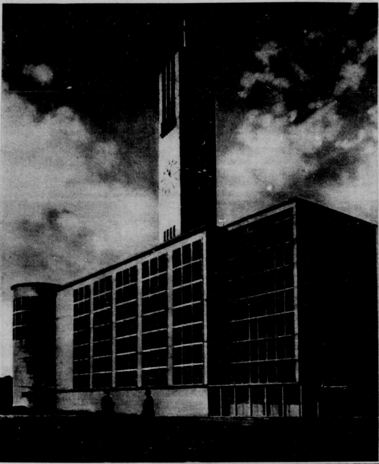
Die erste Eisenbetonkirche Deutschlands Die Petri-Nikolai-Kirche in Dortmund stellt ein Musterbeispiel der modernen Kirchenarchitektur dar. Die Kirche ist ein Betonskelettbau aus schlanen Rahmen. Das Stützensystem rahmt durchsichtige Wände aus leuchtendem Farbglas. (Entwurf: Architekten Finke und Grunb) Arch. The New York Times
