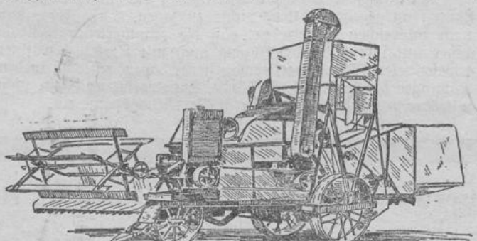
Mährescher, in einem Arbeitsgang mähend und dreschend.
