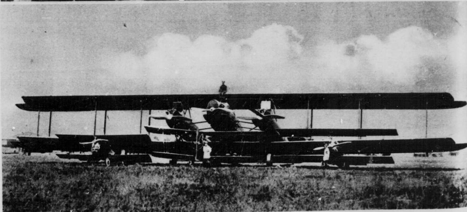
Das größte Bombenflugzeug der Welt im Dienst der amerikanischen Armee Dieses Riesen-Bombenflugzeug ist mit drei Motoren in einer Gesamtleistung von 1500 PS ausgerüstet und hat eine Spannweite von 53 m. Die drei im Vordergrund liegenden Abwehrflugzeuge verdeutlichen die Größe des Bombenflugzeuges, zu dessen Bedienung 6 Mann erforderlich sind. Es erreicht eine Stundengeschwindigkeit von 250 km/h.
