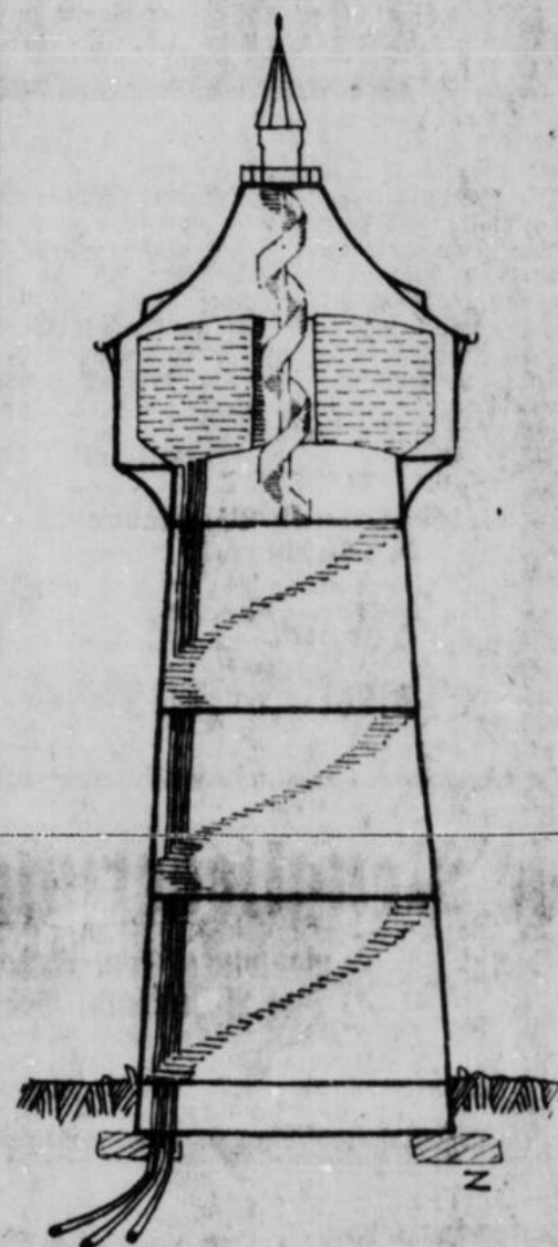
Querschnitt durch einen Wasserturm. Im Innern führen Wendeltreppen in die Höhe.
