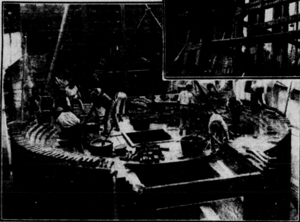
Das gewaltige Fundament des Schornsteins, der die respektable Höhe von 135 m bekommt. Vor dem Bau waren in dem felsigen Boden umfangreiche Sprengungen nötig.
