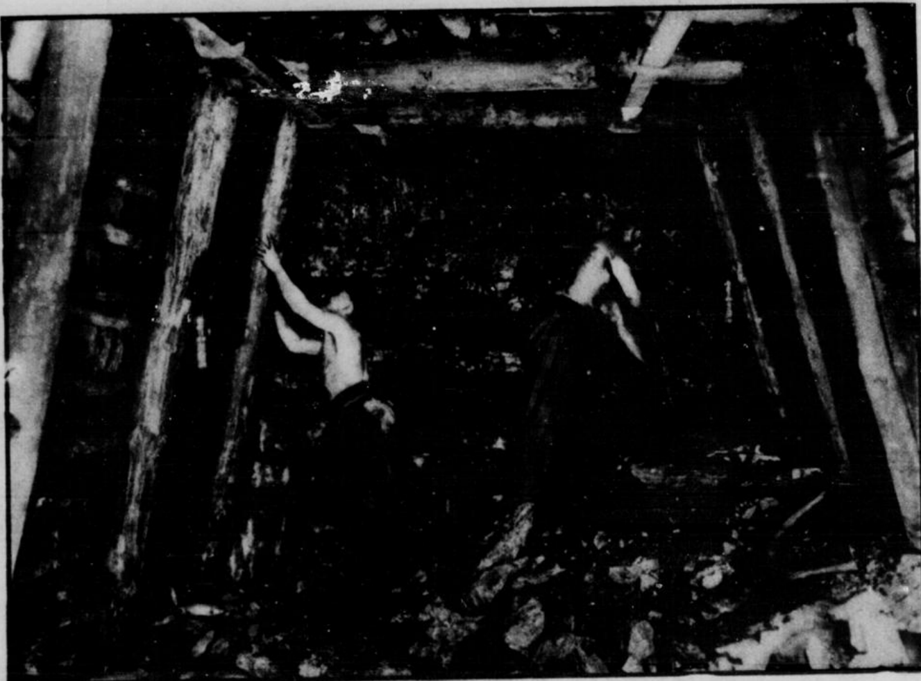
Kohlenhauer vor Ort mit Abbaushammer Links: Schwere Schrämmaschine in Tätigkeit
