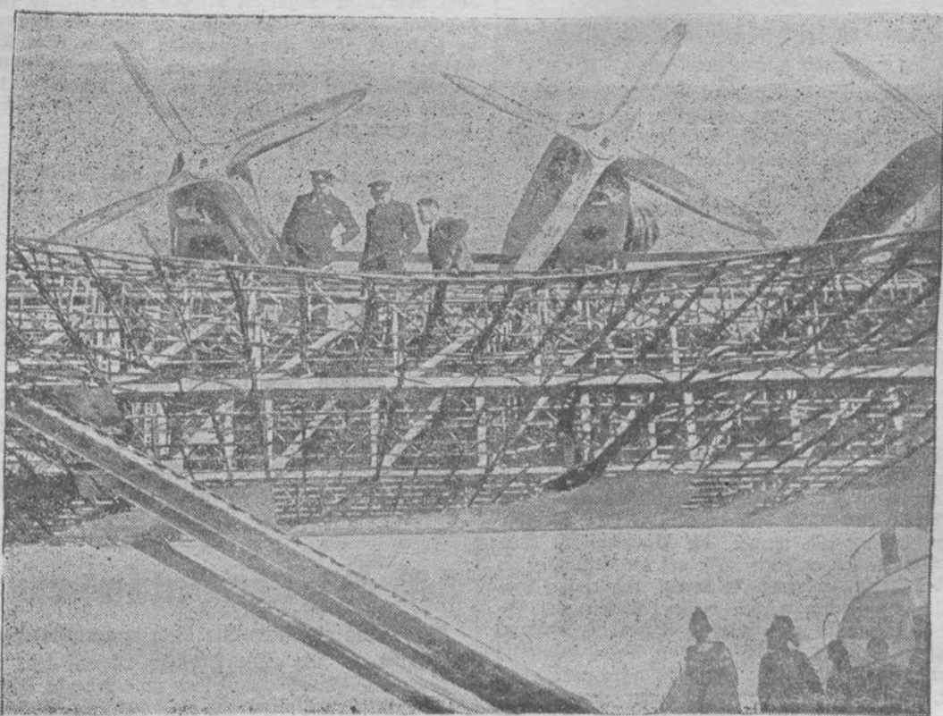
Dieses Metallgerippe blieb übrig von dem linken Flügel des Do X, an dessen Bord im Hafen von Lissabon plötzlich ein Brand ausbrach. An der Aus- besserung des Schadens wird bereits eifrig gearbeitet.
