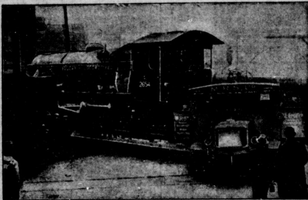
Zum Transport von Lokomotiven aus der Werkstatt zum Hafen, wo sie nach Indien verladen werden, verwendet eine englische Firma diesen Pezomastor. Er ist etwa 20 Meter lang und wird von einem Dieselmotor bewegt.
