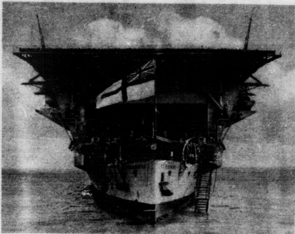
Der englische Flugzeugträger „Glorious“ Bild zeigt den hinteren Teil des Schiffes, wo der überdachte Aufenthaltsraum für die 30 mitgeführten Flugzeuge endet
