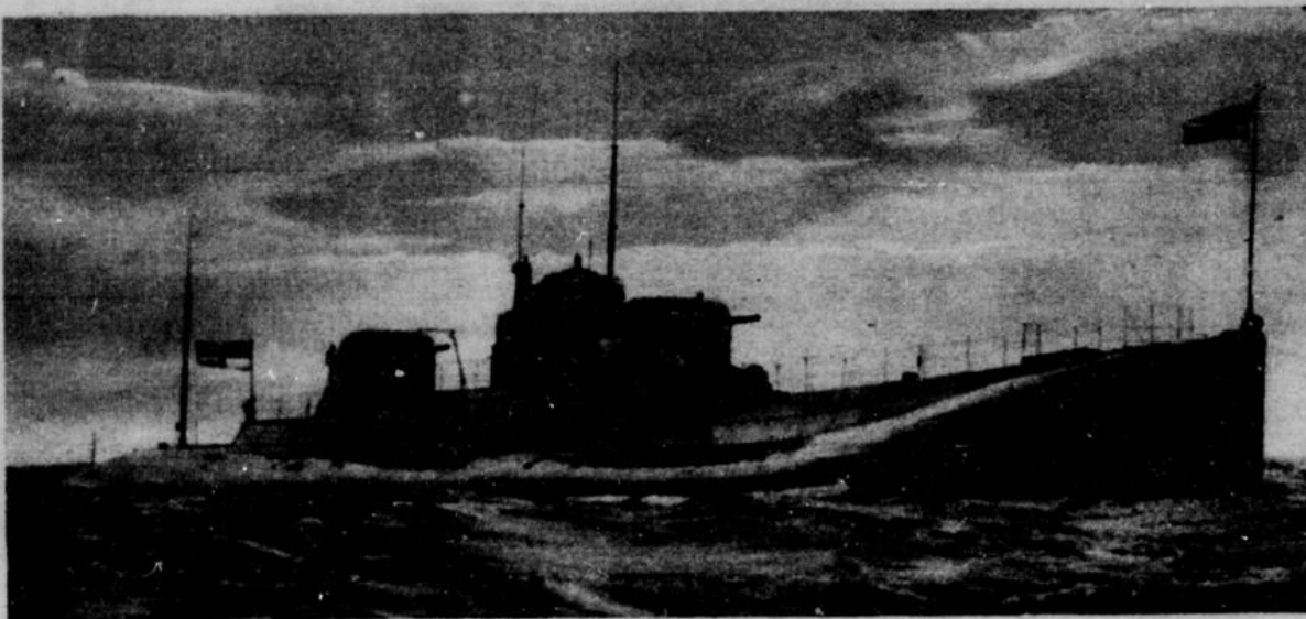
Englisches Groß-U-Boot X 1 Wasserverdrängung: 3600 Tonnen. Länge: 121 m. Armierung: 4 15-cm-Geschütze. 6 Torpedorohre. Besatzung 121 Mann Aut. H. Wolff-Transatlantische
