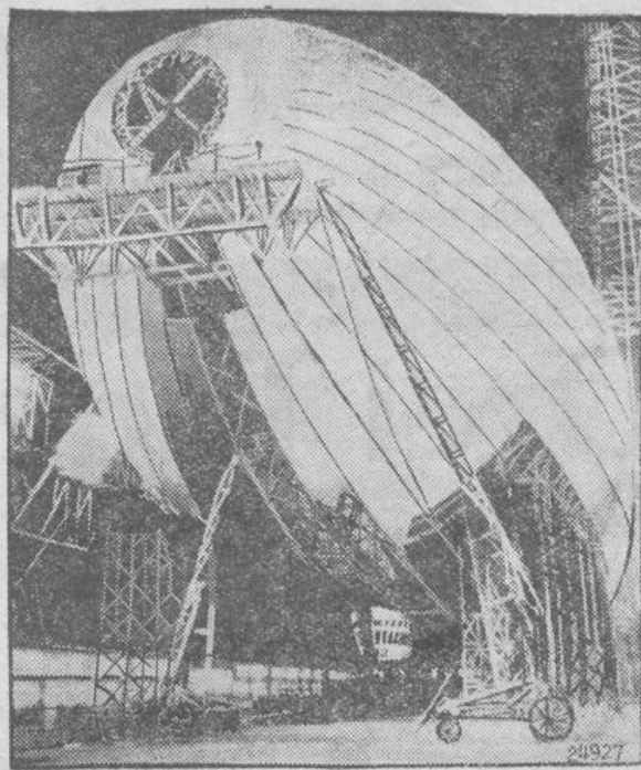
Der Welt größtes Luftschiff vor der Vollendung. Das Marineluftschiff „Akron“, das zur Zeit in Akron (Ohio) gebaut wird, ist nahezu fertiggestellt, und wird demnächst seine ersten Probeflüge unternehmen.
