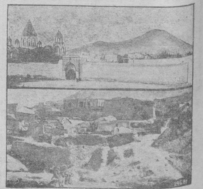
Das Erdbeben im Kaukasus.
