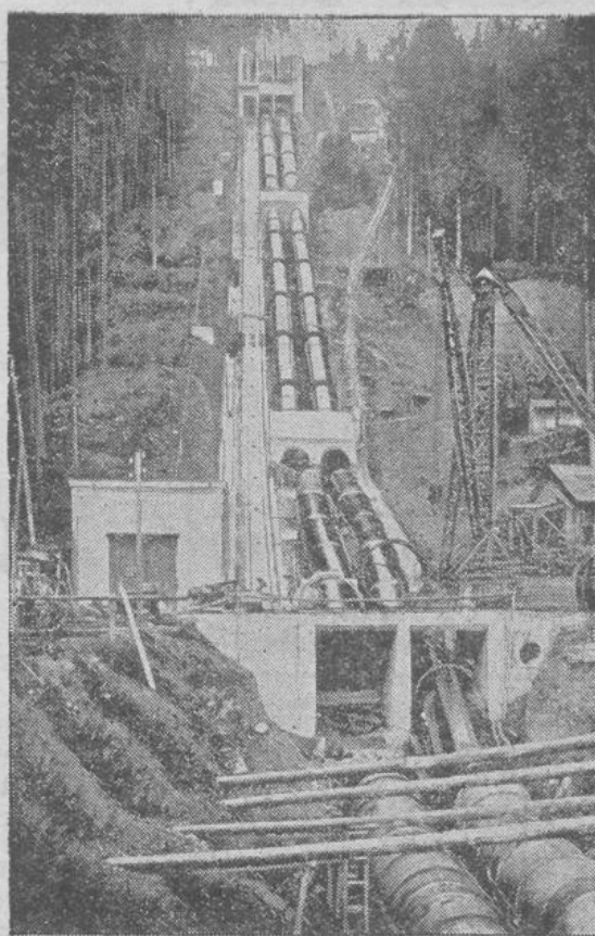
Neues deutsches Großkraftwerk im Bau.
