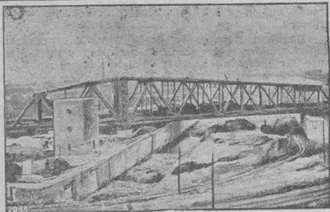
Die Schwebel-Drehbrücke der Welt. Als ein Bestandteil der Norddeutschen Anlage in Bremerhaven wurde diese 115 Meter lange und 19 Meter breite ungleichermaßen Drehbrücke errichtet. Sie verbindet die Fahrgastanlagen am Columbusstai mit dem Hinterland. Das Gesamtgewicht der Brücke beträgt 2700 T. Elektromotorische Antriebsmaschinen ermöglichen es, die Brücke in 3 Minuten ein- oder auszufahren.
