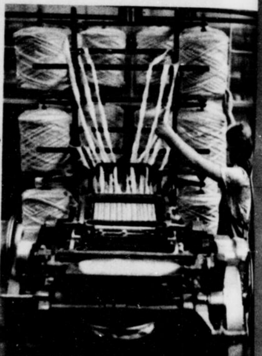
Nachdem die gewaschene flaumige Masse über beheizte Walzen und durch diesen Kämmprozess in die enge Bandform, eine sogenannte „Fließ“, gebracht wurde, wird sich hier in feinen bezahnten Kammmaschinen der Fadenzug weiter
