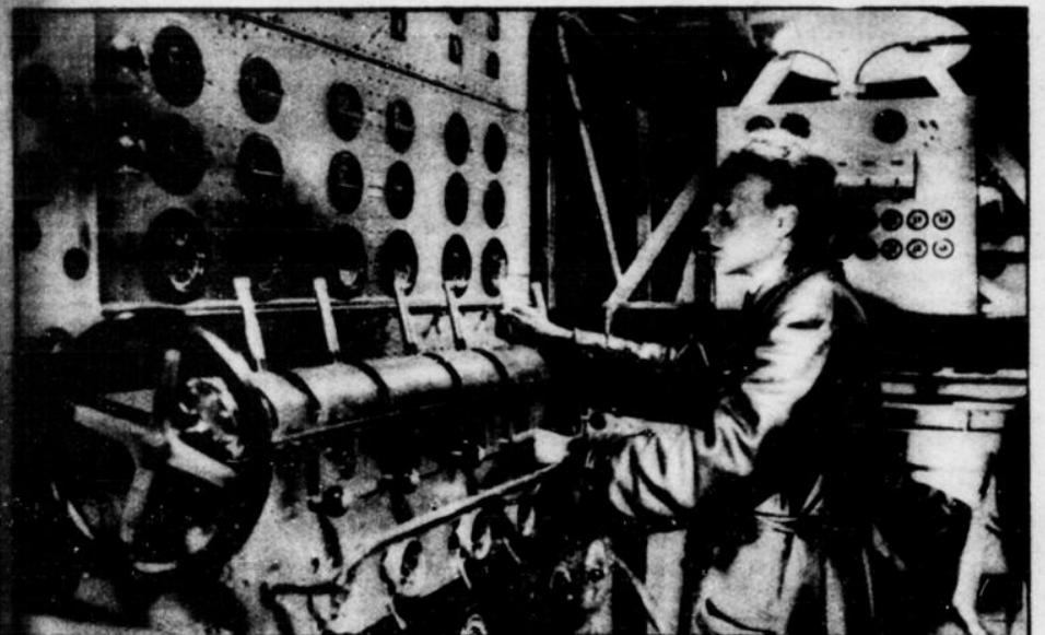
Das Herz des Riesen-Flugbootes „Do. X“, Maschinenzentrale und Kommandoraum, von dem aus die 12 Motoren geleitet werden
