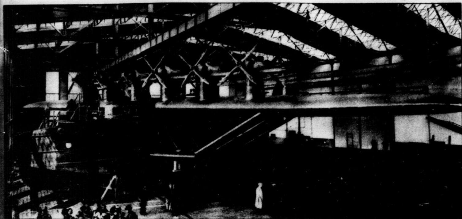
Das größte Flugschiff der Welt, das Dornier-Flugschiff „Do. X“, nach seiner Fertigstellung in der Halle der Dornier-Werft in Altenrhein am Bodensee
