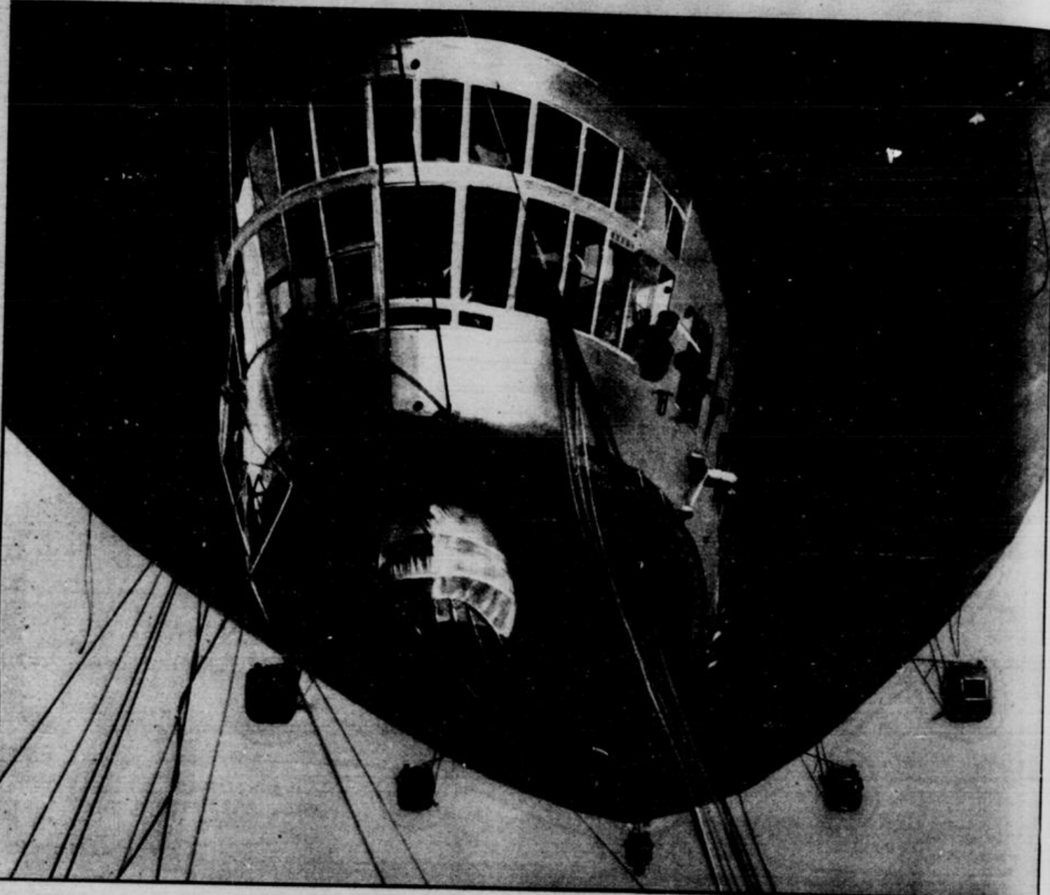
Blick auf die große Führergondel und die fünf Maybach-Motoren am Rumpf des Luftschiffes „Graf Zeppelin“.
