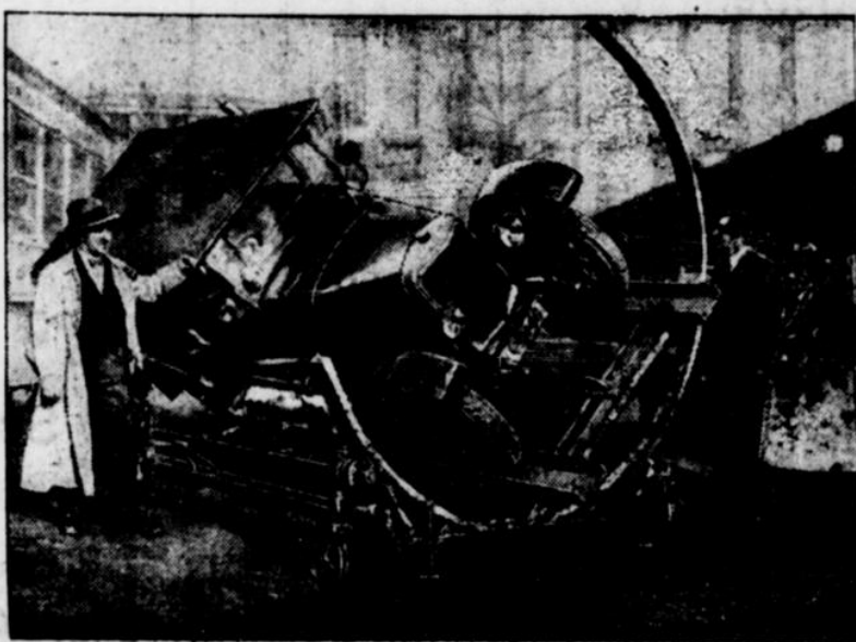
Eine neuartige Kippvorrichtung für Autoreparatur-Werkstätten. Das Auto fährt auf Schienen auf die Kippvorrichtung und wird dann durch eine Handturbel in die gewünschte Lage gebracht.
