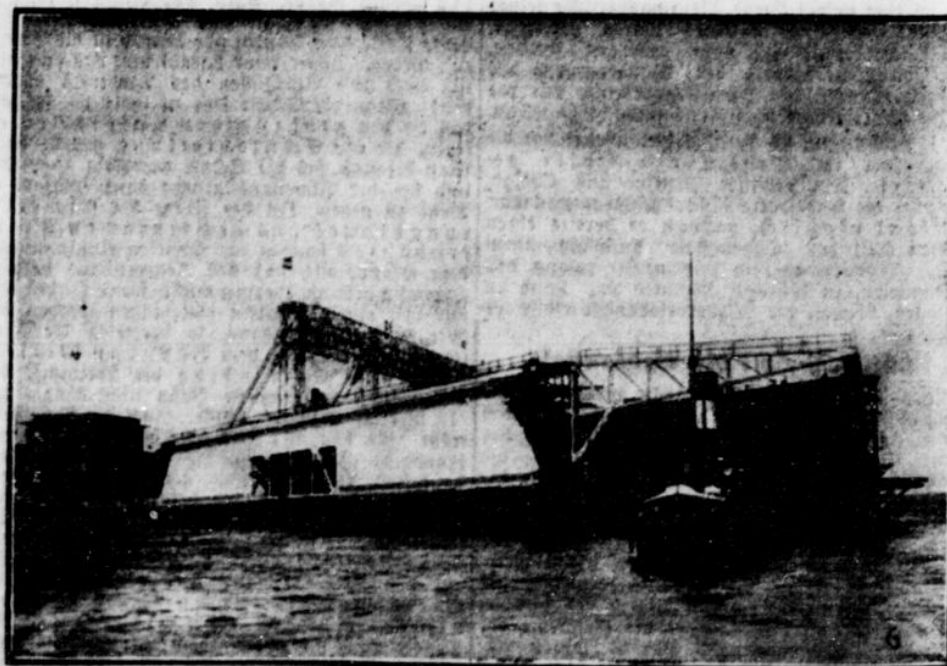
Das zweite auf Reparationskonto gebaute Schwimmdock für den Hafen von Rouen wurde bei der Deutschen Werft in Hamburg vom Stapel gelassen.
