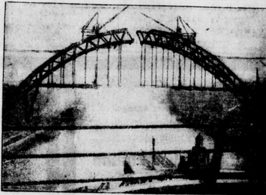
Die beiden Teile der neuen Hochbrücke über den Dyne bei New-Castle, die den Fluß in einem Bogen von 200 Metern Spannweite überbrückt, und deren Fahrbahn so hoch liegt, daß sogar große Seeschiffe unter ihr durchfahren können.
