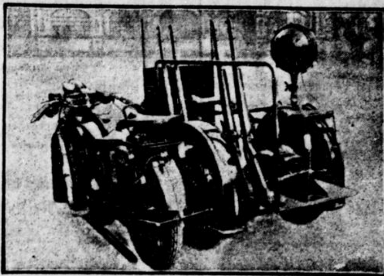
Bei der Berliner Schuppolizei werden zurzeit Versuche mit einem neuartigen Erreife-Fahrzeug durchgeführt, das aus einem Motorrad mit zweirädriger Seitenwagen besteht und auf dem außer dem Fahrer vier Schutzleute Platz haben.
